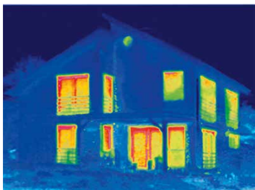
Infrarotaufnahmen, Thermografien, zeigen deutlich, wo ein Haus unkontrolliert Energie verliert. Rot bedeutet Wärme und damit hohen Energieverlust.
